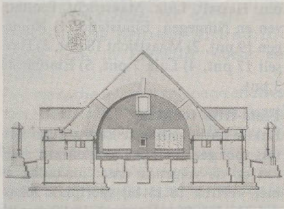
Doorsnee-tekening van standaard ontwerp voor een kruithuis.
