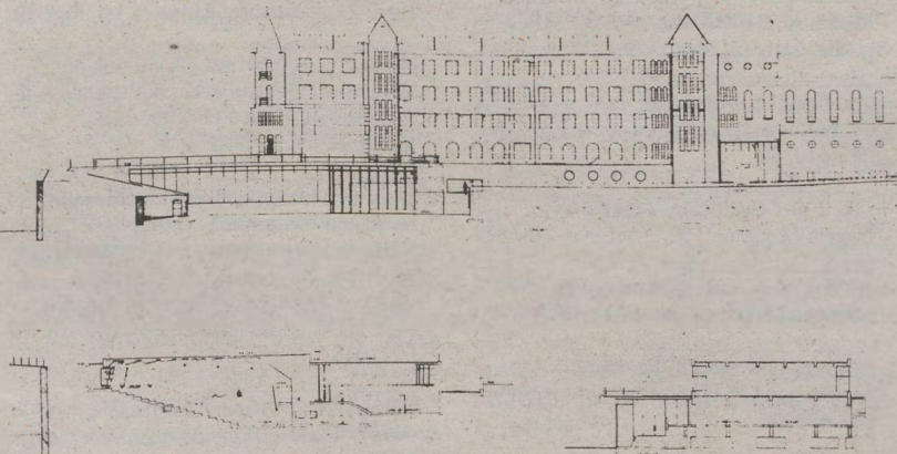
Zij-aanzicht van Tongersestraat 53 met links de stadswal en rechts de Tongersestraat. Op de onderste tekeningen links een doorsnee van de collegezaal en rechts van de nieuwe zij-ingang
